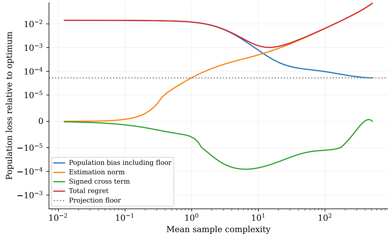
rich6d: T=7290
